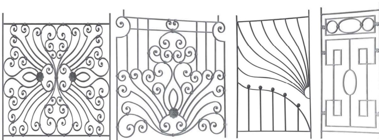
Q12 1000x1185 Q12 1000x970 ≠20x6 1000x670 ≠14x8 1000x495 GD239/1 GD236/1 GD247/1 GD205/1
