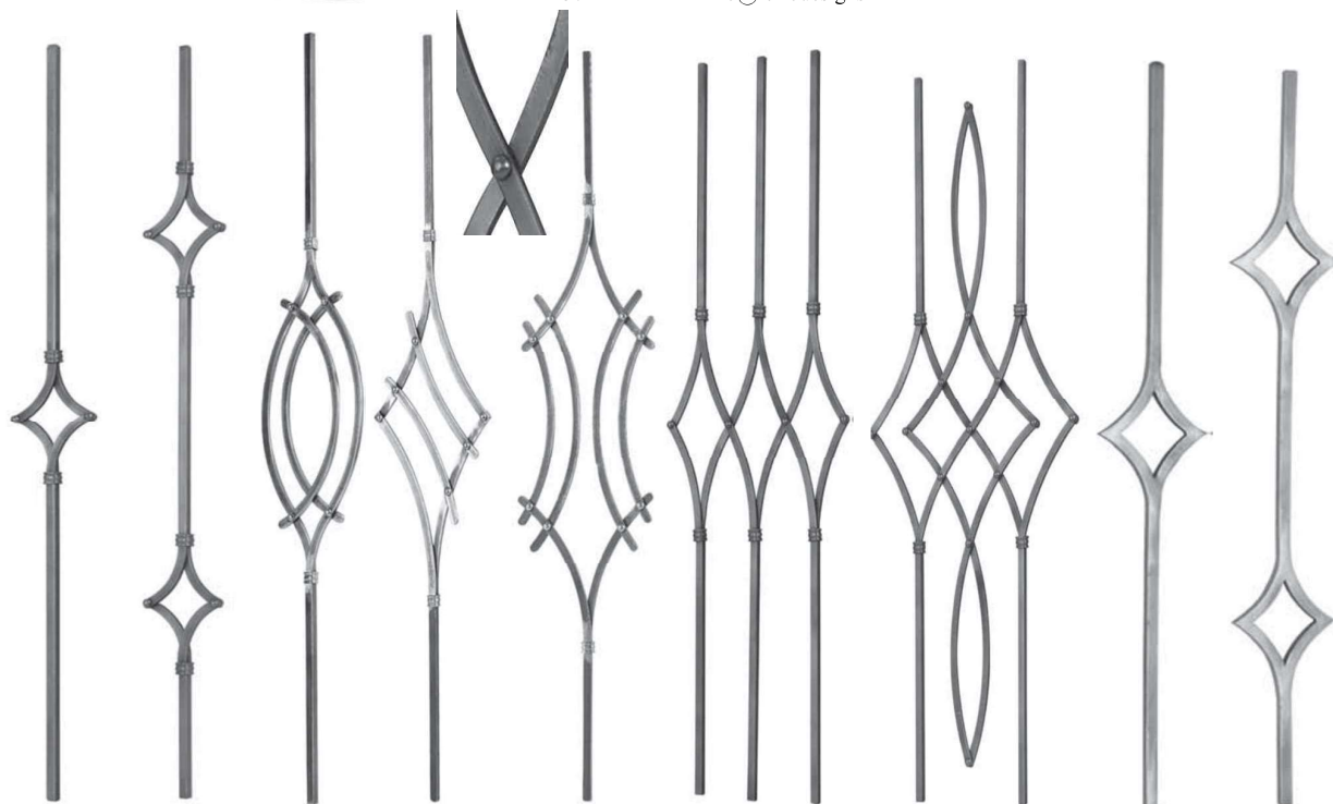
Q12 Q12 Q12 Q12 Q12 Q12 Q12 Q12 Q12 1000x110 1000x110 1000x180 1000x200 1000x200 1000x315 1000x345 1000x120 1000x120 GD20/1 GD20/2 GD20/5 GD20/8 GD21/3 GD21/1 GD21/2 GD58/3 GD58/2
